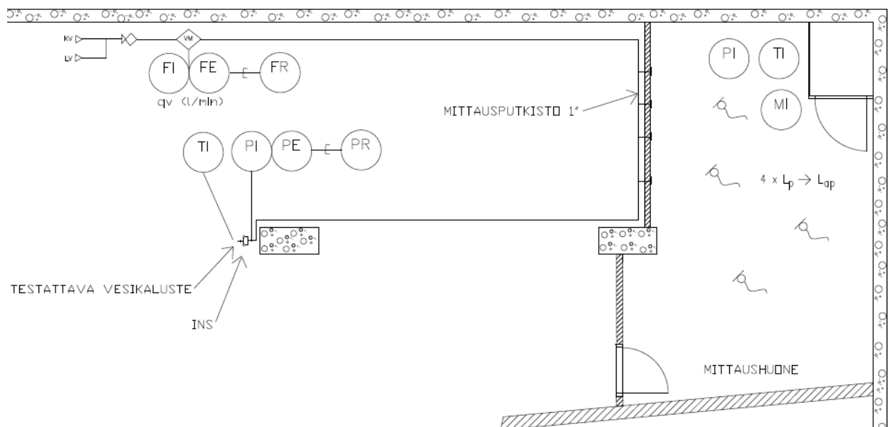
Kuva 2. Mittausperiaate vesikalustemelutasomittauksissa.
