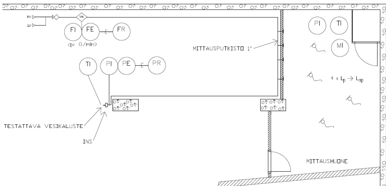
Kuva 2. Mittausperiaate vesikalustemelutasomittauksissa.
